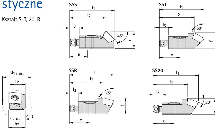
Rysunki narzędzi w wersji prawej – przykład SSR.
