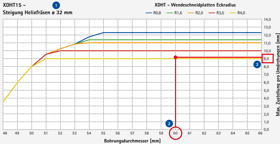
XDHT15 – Steigung Helixfräsen \varnothing 32 mm
