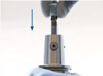
信息： 为了正确夹紧刀具，刀具的HB-面必须朝向夹紧螺钉对准。 2. 将刀具包括刀柄向前推入侧固式刀柄的装夹孔。 刀具上的凹槽指向夹紧螺钉。
