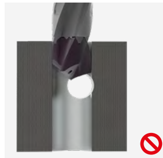
Otwór niecentryczny; ścin poza kontaktem ze ścianą otworu
