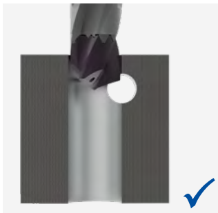
Otwór niecentryczny; ścin w kontakcie ze ścianą otworu
