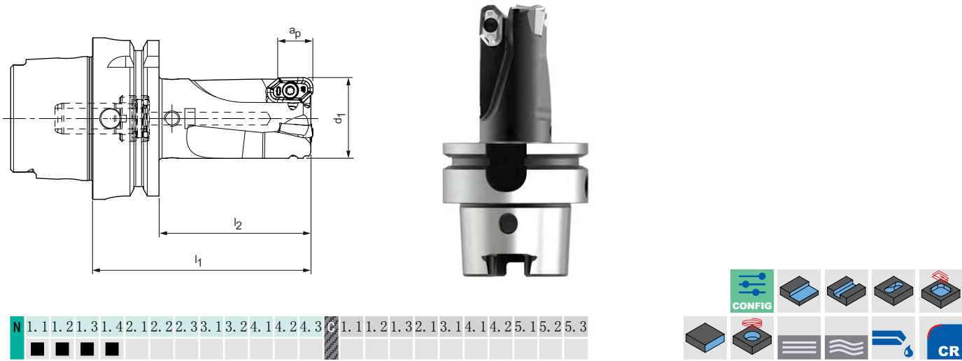
可配置系列尺寸 | 带有 HSK-A63 链接尺寸
