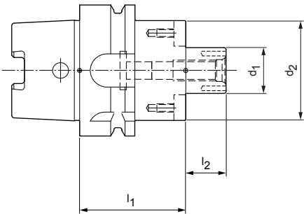
HSK-A 刀柄带有分散式冷却剂供给 | 可应要求提供
