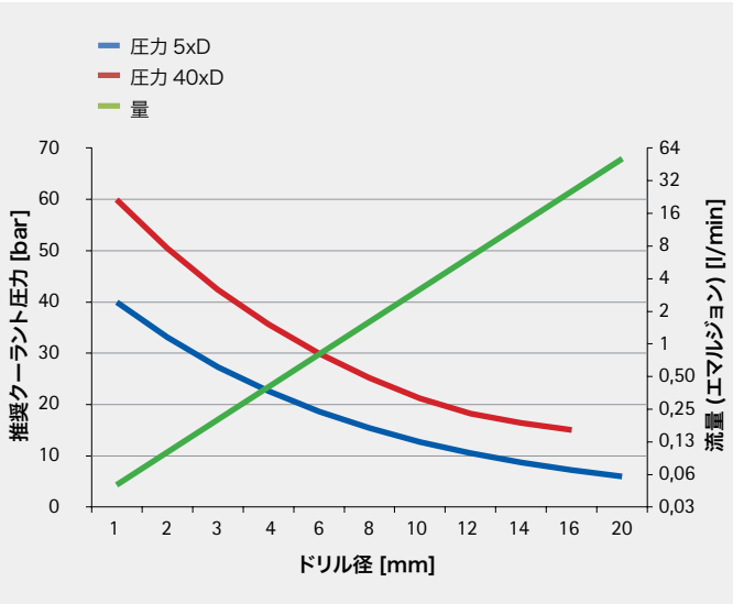
クーラント圧および量の基準値
