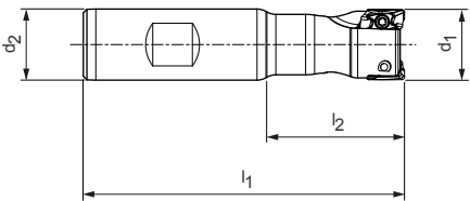
立铣刀
