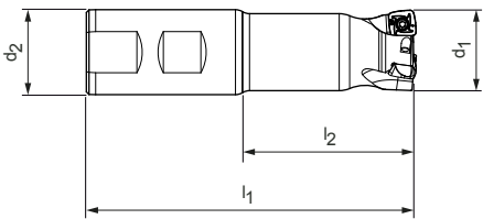
立铣刀
