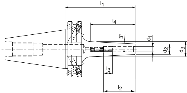
细长结构形式 3°
