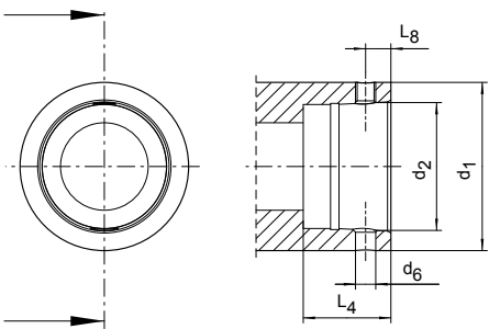
HSK-E 用于手动换刀
