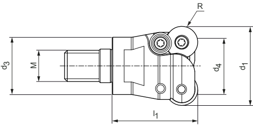
螺纹连接铣刀，圆柱结构形式
