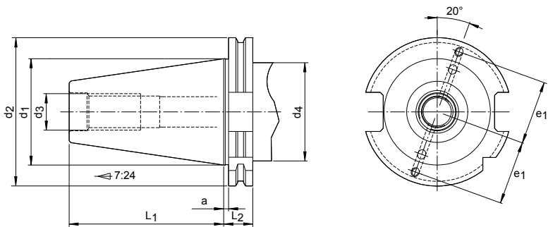
用于自动换刀A型、AD型、AF型和带数据芯片的结构形式
