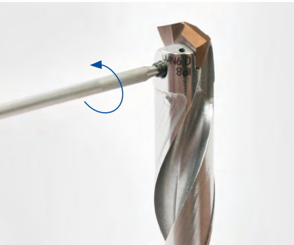
1. 借助随附的TORX® PLUS扳手以逆时针方向转动，松开专用夹紧螺钉。
