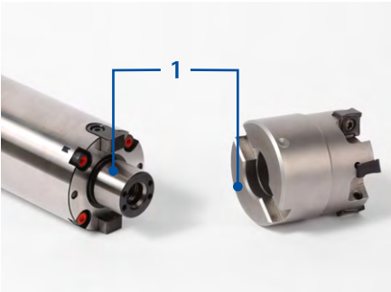
1. 清洁套式铣刀刀柄和刀具（1）的装夹区域。
