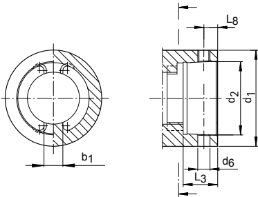
HSK-C 用于手动换刀
