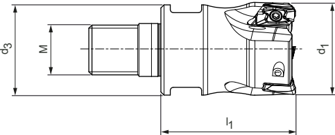
螺纹连接铣刀
