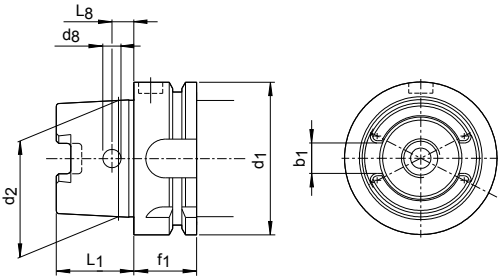
HSK-A 用于自动和手动更换刀具
