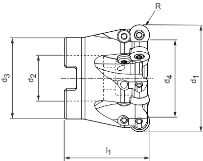
铣刀盘
