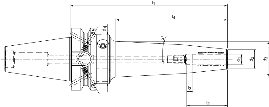
细长结构形式 3°，优化轮廓用于获得最大抗弯刚度
