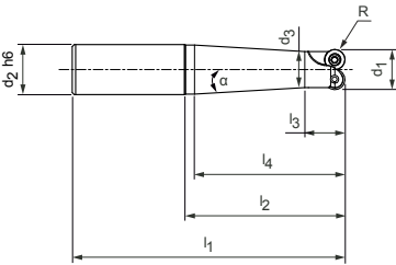
立铣刀，锥形结构形式
