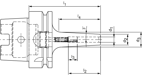
细长结构形式3°
