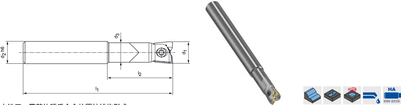
立铣刀，带整体硬质合金的圆柱结构形式
