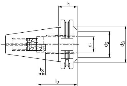
超短型结构形式
