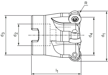
铣刀盘
