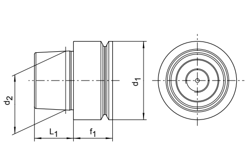
HSK-E 用于自动换刀
