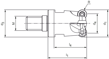
螺纹连接铣刀，锥形结构形式
