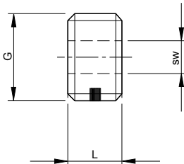
螺堵
