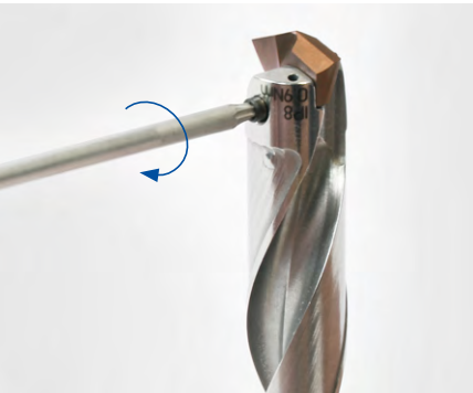
4. 将新刀片放入刀片座中。借助随附的TORX® PLUS扳手以顺时针方向拧紧专用夹紧螺钉。
