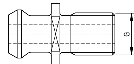
用于长锥柄的拉钉 符合 ASME B 5.50 (CAT)
