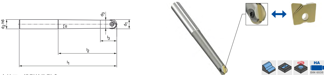
立铣刀，锥形结构形式
