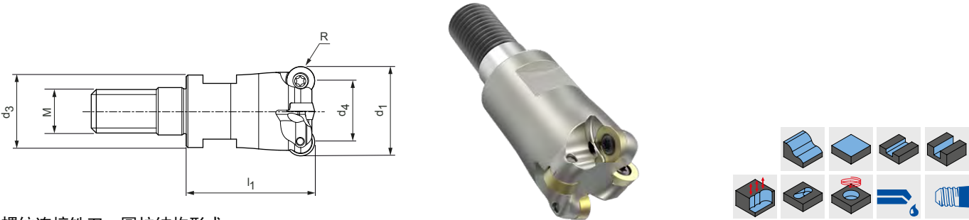
螺纹连接铣刀，圆柱结构形式
