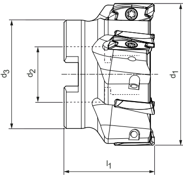
铣刀盘
