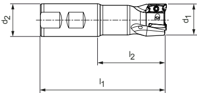
立铣刀
