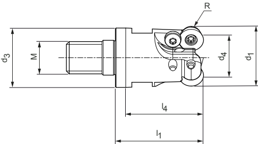
螺纹连接铣刀，锥形结构形式
