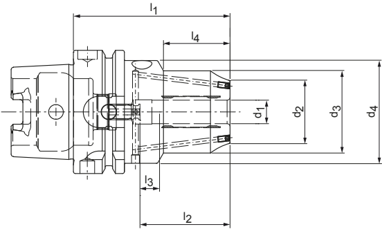
短重型结构形式带两个冷却通道孔，可重新封闭
