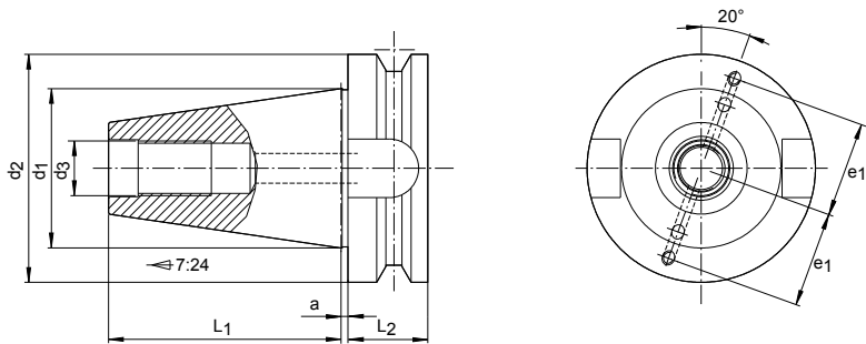
用于自动换刀 J型、JF型、JD型和带数据芯片的结构形式
