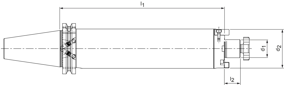
减振结构
