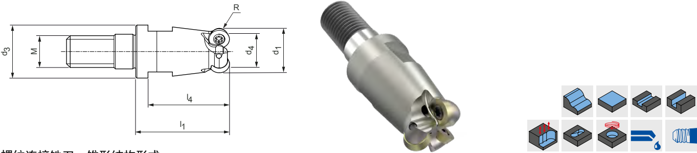
螺纹连接铣刀，锥形结构形式
