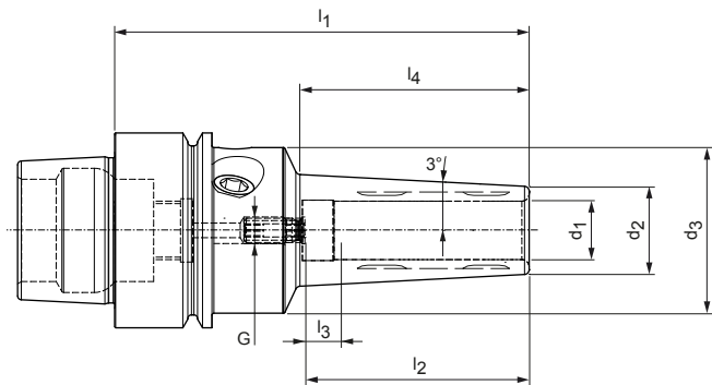
细长结构形式 3° | 可应要求提供
