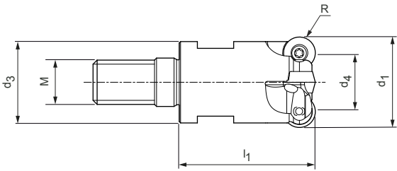
螺纹连接铣刀，圆柱结构形式
