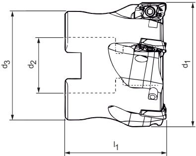
铣刀盘
