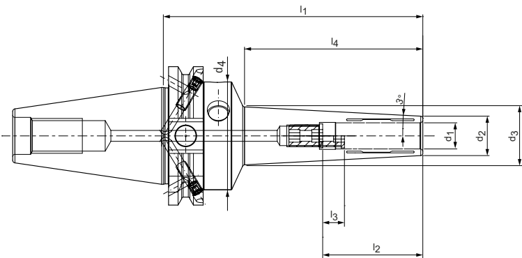
细长结构形式 3°
