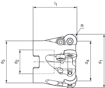
铣刀盘
