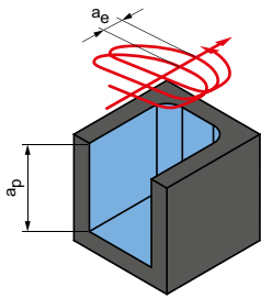
摆线 铣削
