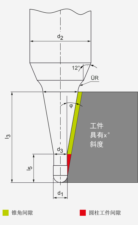
插图 2：锥角和颈部阶梯
