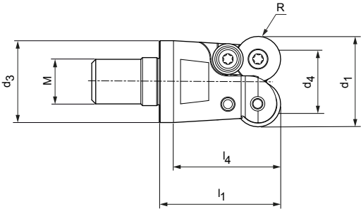
螺纹连接铣刀，锥形结构形式
