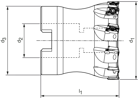
铣刀盘
