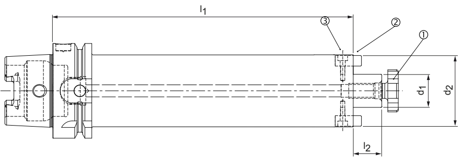
符合DIN 69882-3标准，用于带加大的夹紧端面直径的铣刀刀柄
