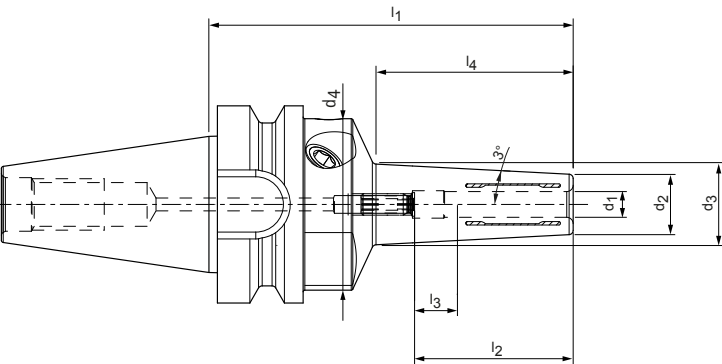
细长结构形式 3°
