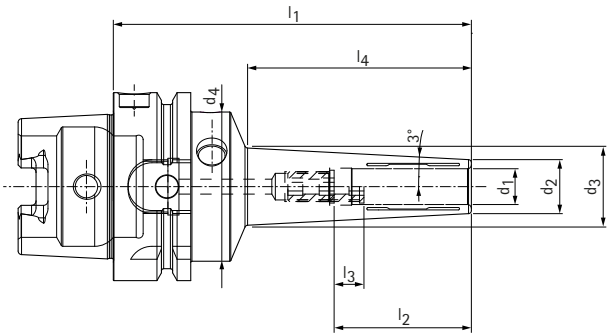
细长结构形式 3°
