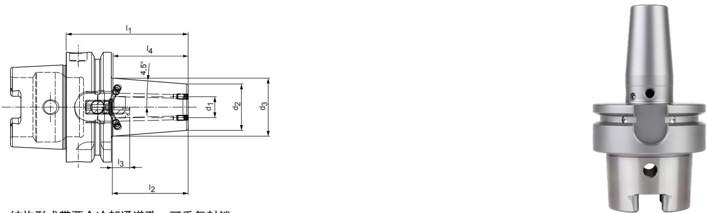
结构形式带两个冷却通道孔，可重复封锁
