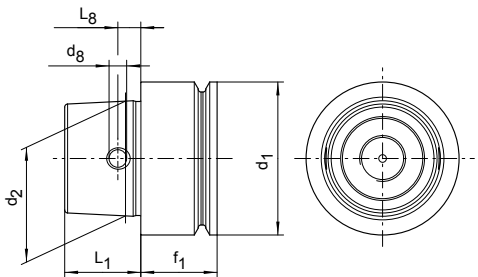
HSK-E 用于自动和手动更换刀具
