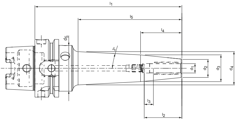
细长结构形式 3°，优化轮廓用于获得最大抗弯刚度
