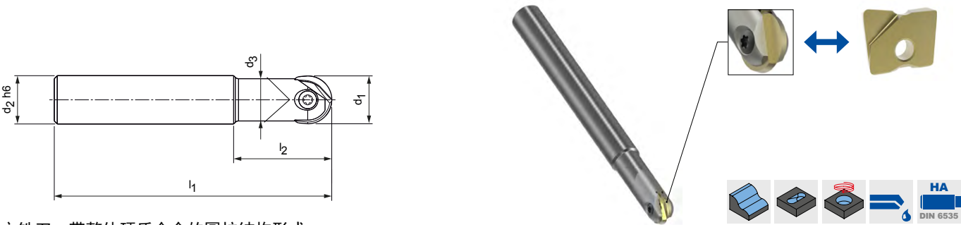
立铣刀，带整体硬质合金的圆柱结构形式
