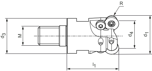
螺纹连接铣刀，圆柱结构形式
