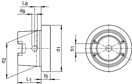
HSK-C 用于手动换刀
